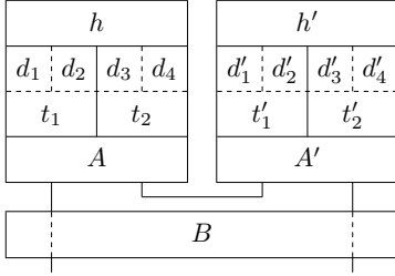
Fig. 1. Example HRAM net
